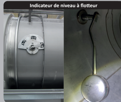
Indicateur de niveau à flotteur
