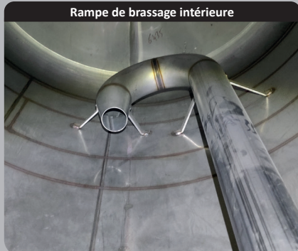
Rampe de brassage intérieure
